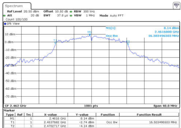
11G-Ant1-2462
