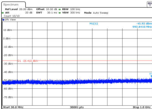
11G-Ant1-2412-30~1000-PASS
