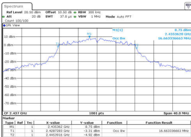
11G-Ant1-2437
