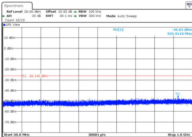
11G-Ant1-2462-30~1000-PASS
