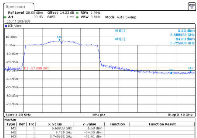
11AC80SISO-Ant1-5610-PASS
