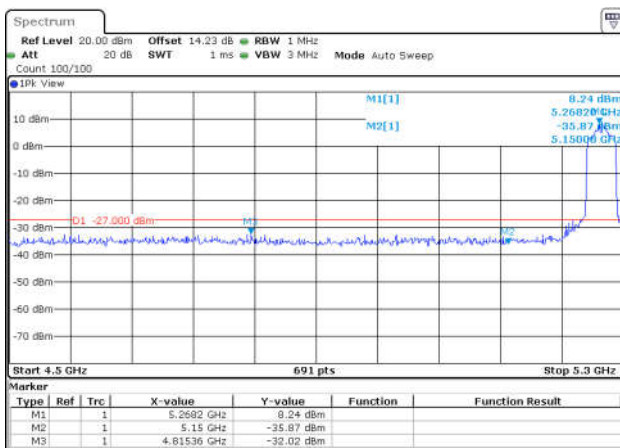
11N40SISO-Ant1-5270-PASS
