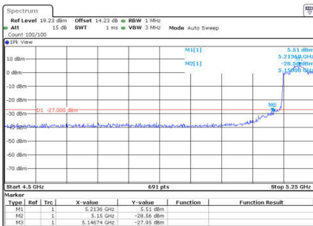
11AC80SISO-Ant1-5210-PASS
