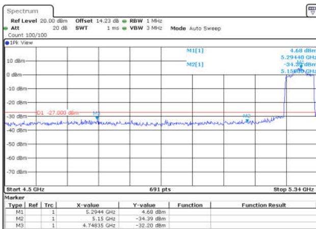
11AC80SISO-Ant1-5290-PASS
