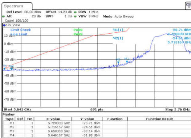
11N40SISO-Ant1-5755-PASS
