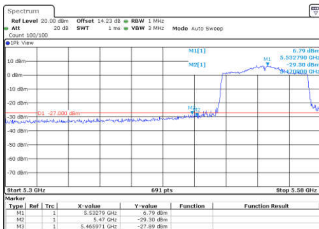
11AC80SISO-Ant1-5530-PASS
