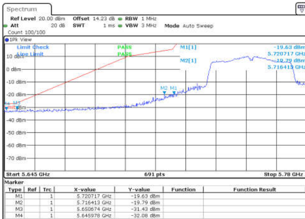
11N40SISO-Ant1-5755-PASS
