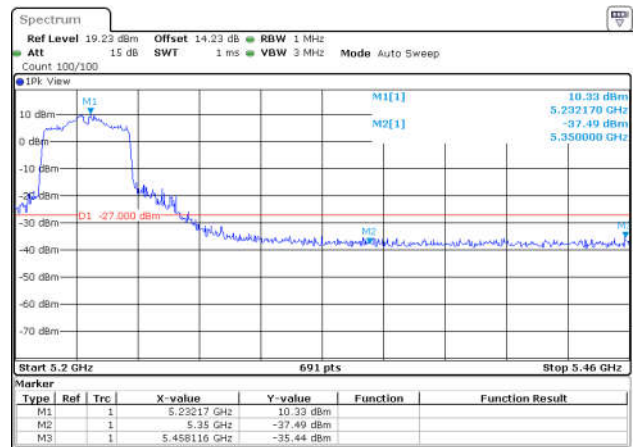
11AC80SISO-Ant1-5210-PASS
