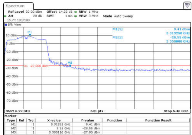
11AC80SISO-Ant1-5290-PASS
