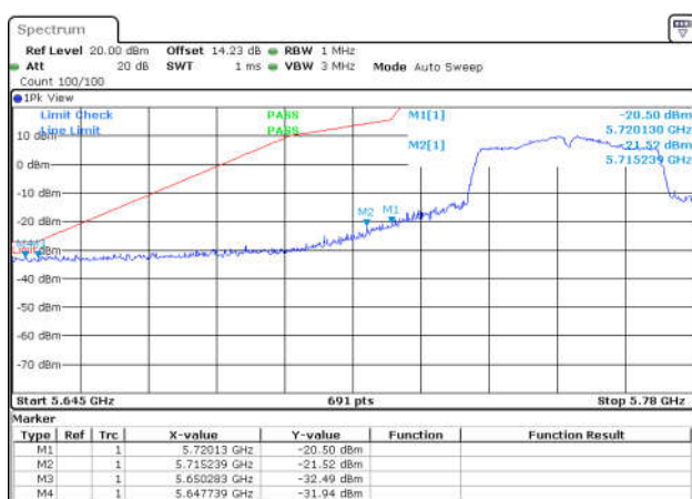
11AC80SISO-Ant1-5775-PASS
