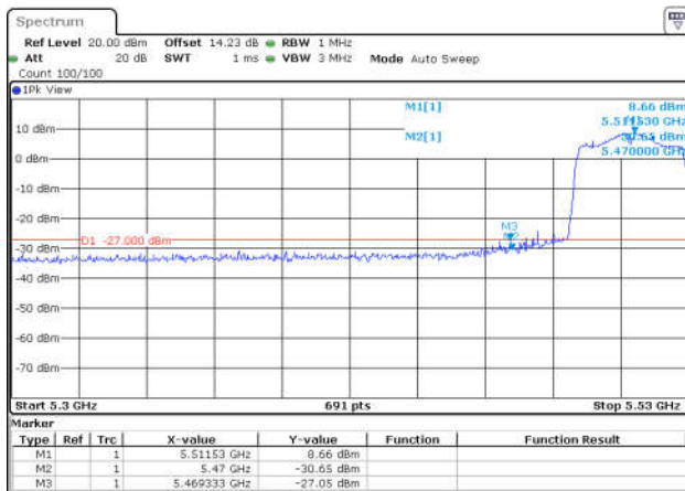
11AC80SISO-Ant1-5530-PASS
