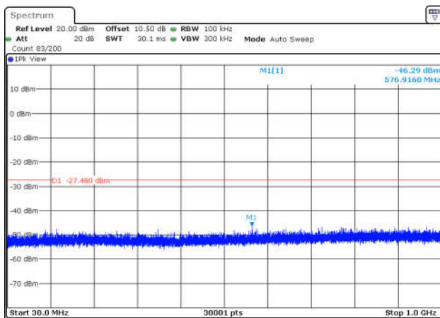
BLE_2M-Ant1-2402-30~1000-PASS
