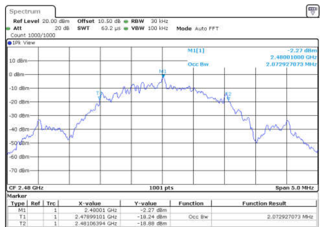
BLE_2M-Ant1-2480
