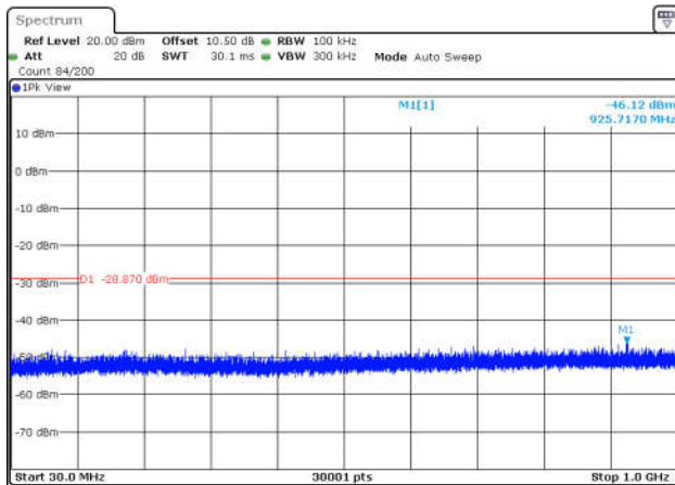
BLE_2M-Ant1-2480-30~1000-PASS
