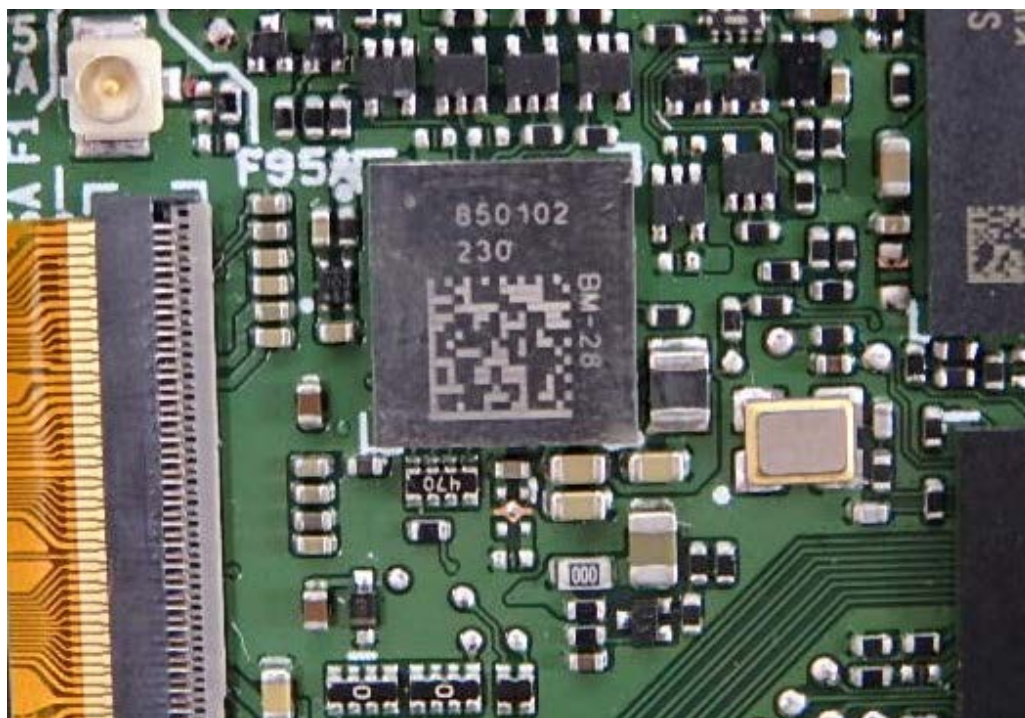
BT&WLAN IC
