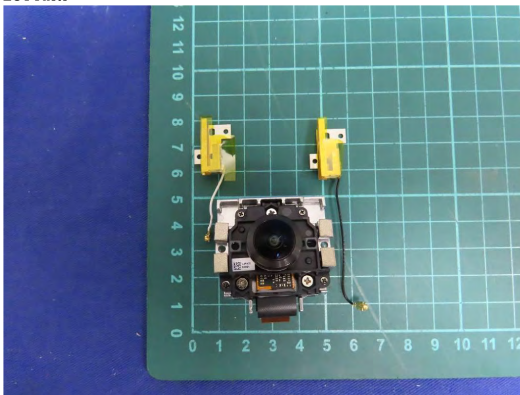
(31) EUT Photo
