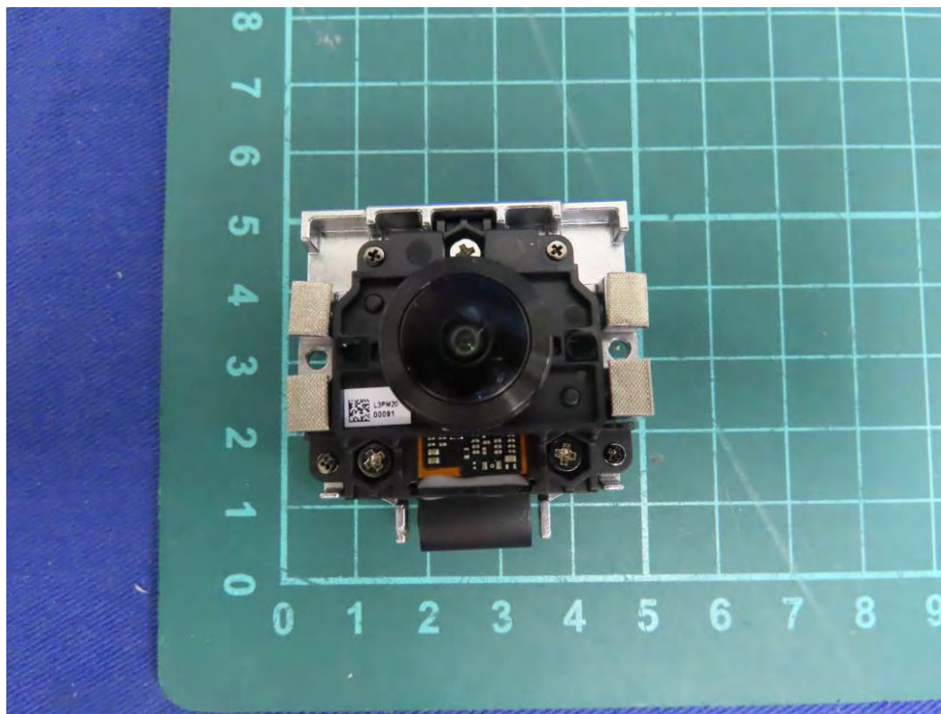
(36) EUT Photo
