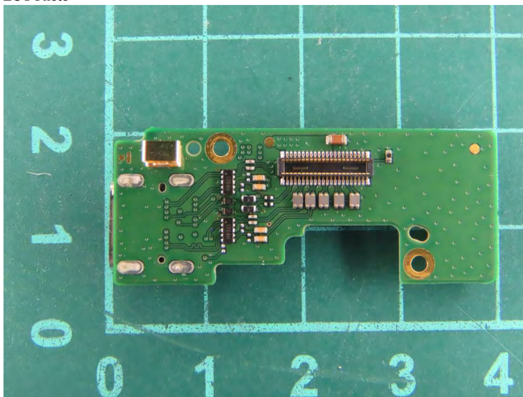
(44) EUT Photo
