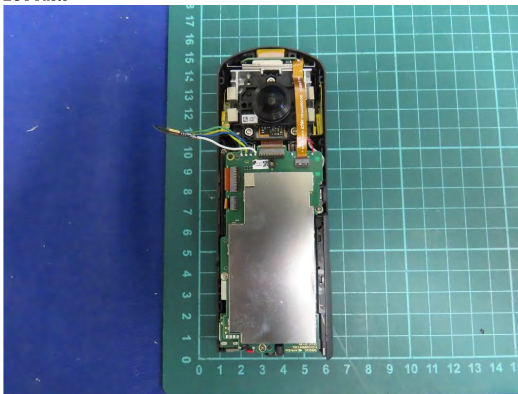
(10) EUT Photo
