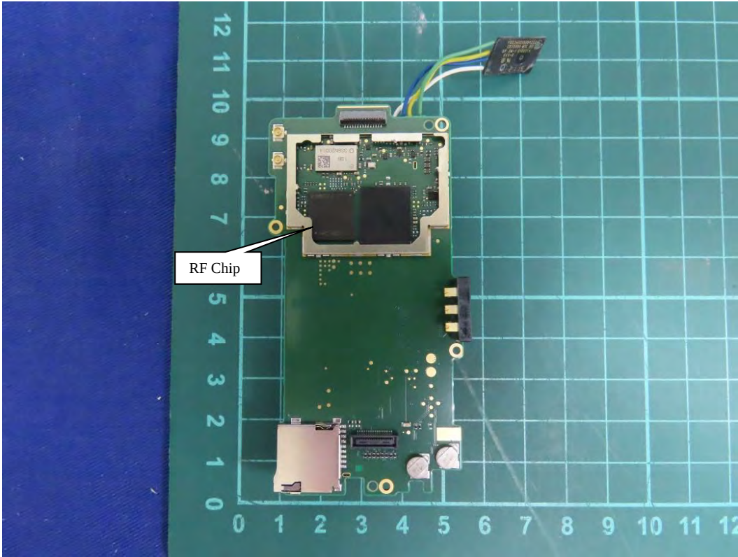
(19) EUT Photo(Antenna)
