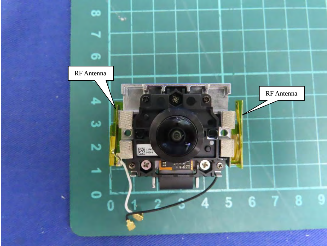
(30) EUT Photo
