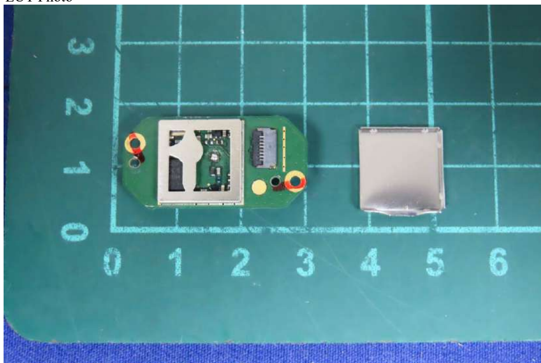
(72) EUT Photo
