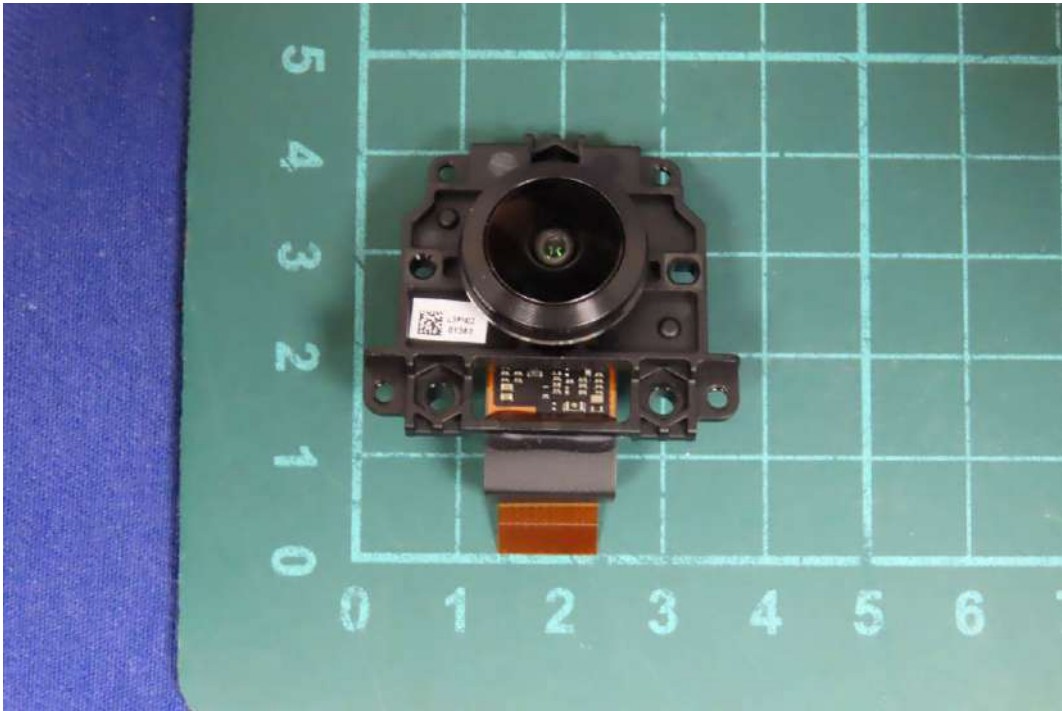
(85) EUT Photo
