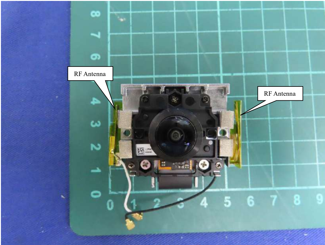
(37) EUT Photo
