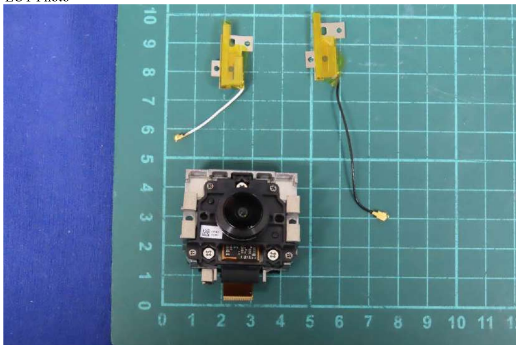
(78) EUT Photo
