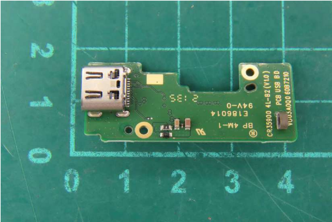
(92) EUT Photo
