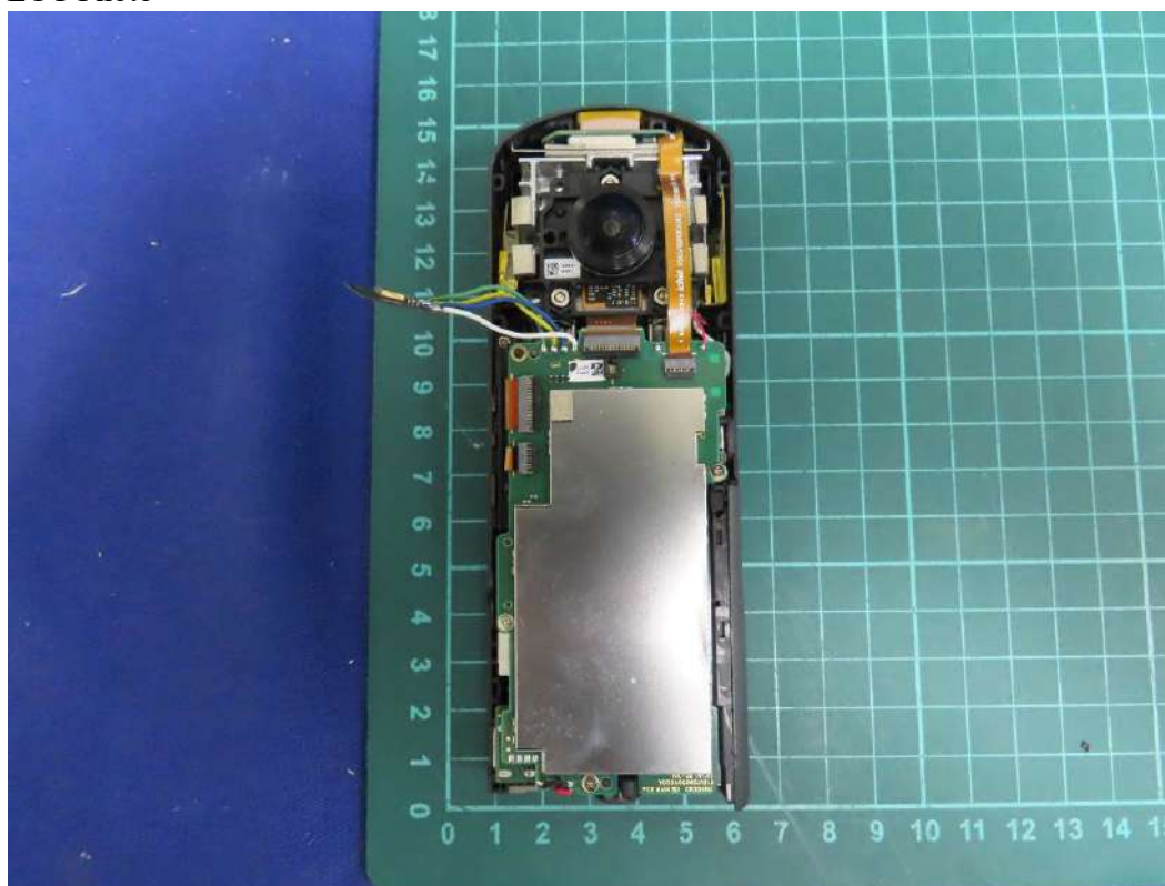
(17) EUT Photo
