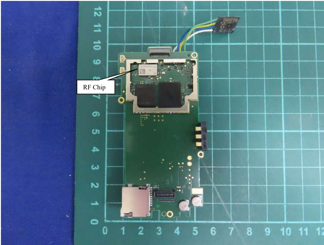
(26) EUT Photo(Antenna)
