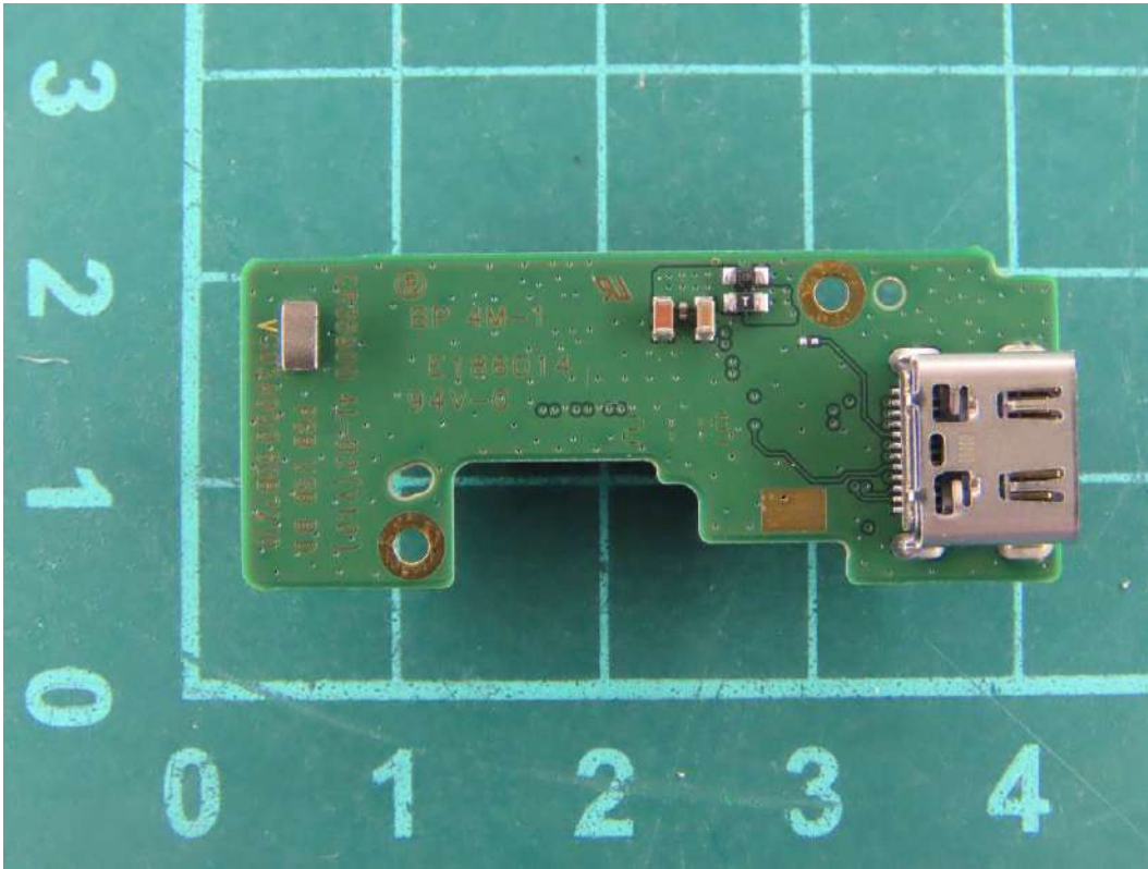
(52) EUT Photo
