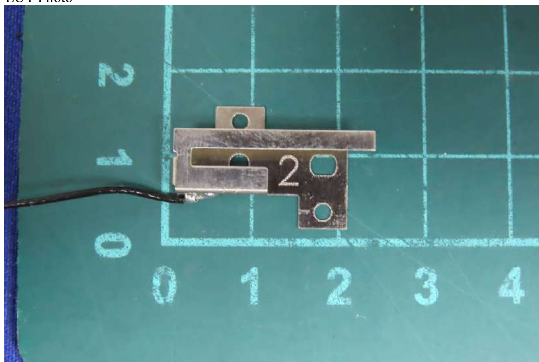
(81) EUT Photo
