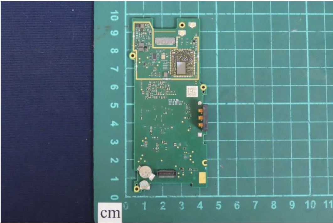
(18) EUT Photo
