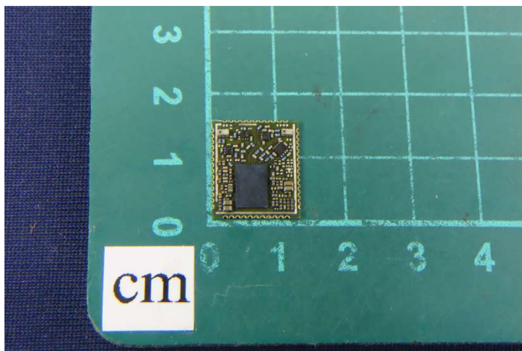
(20) EUT Photo
