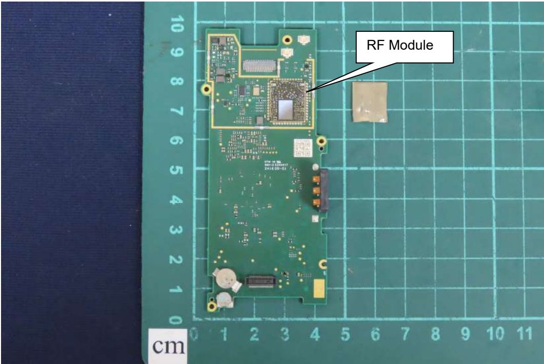
(17) EUT Photo
