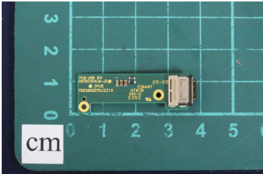
(10) EUT Photo
