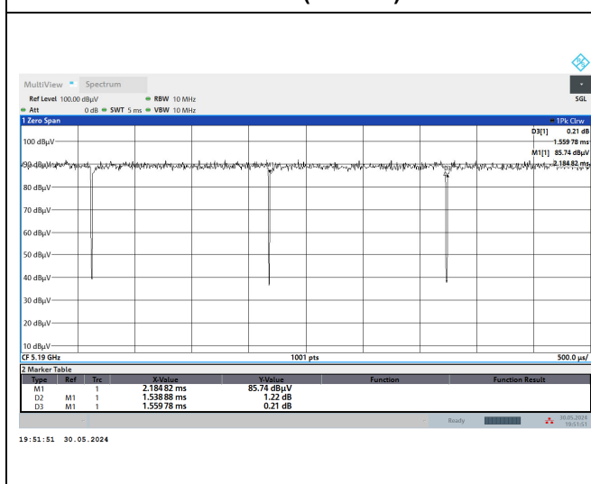
802.11n (40 MHz)
