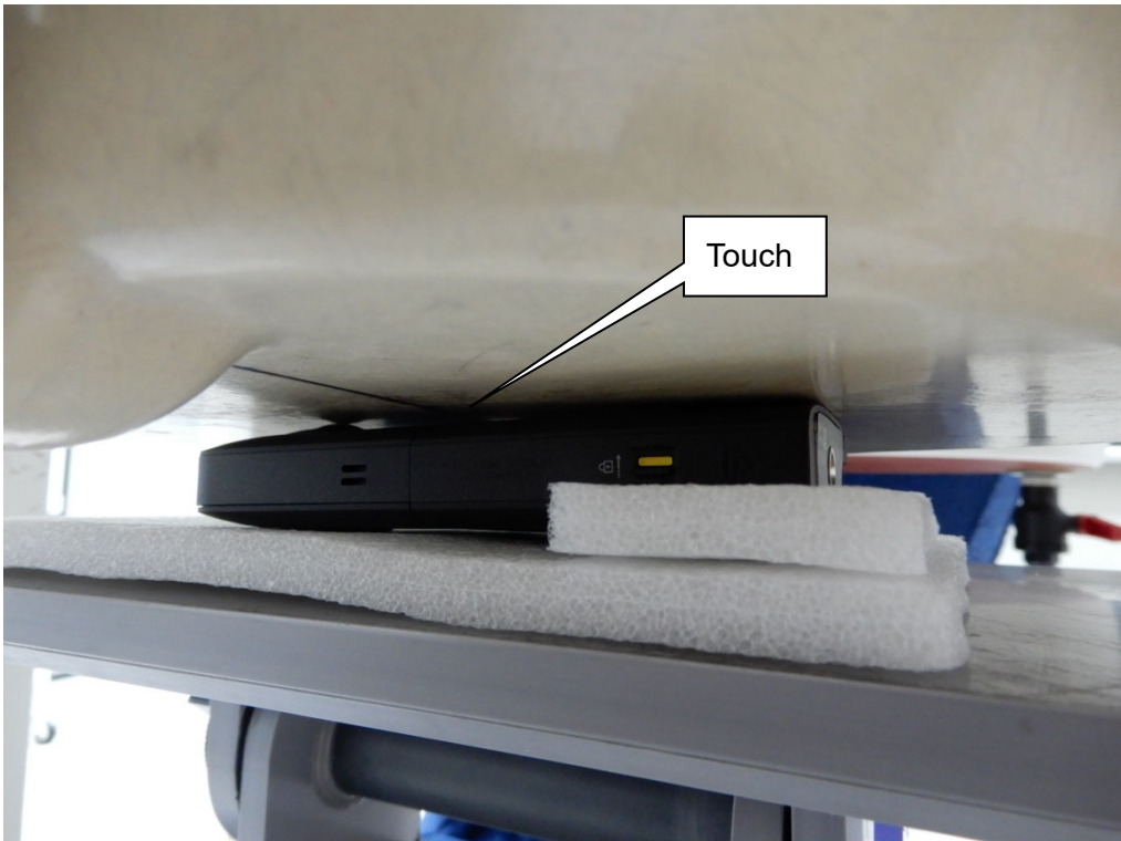
EUT Front
