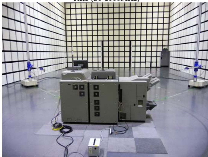
Rear (30-1000MHz)
