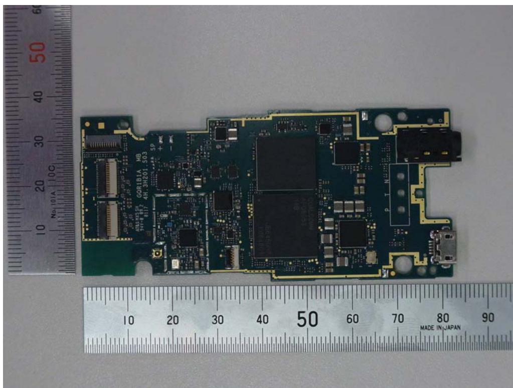
MAIN_top_RF_cover_less
