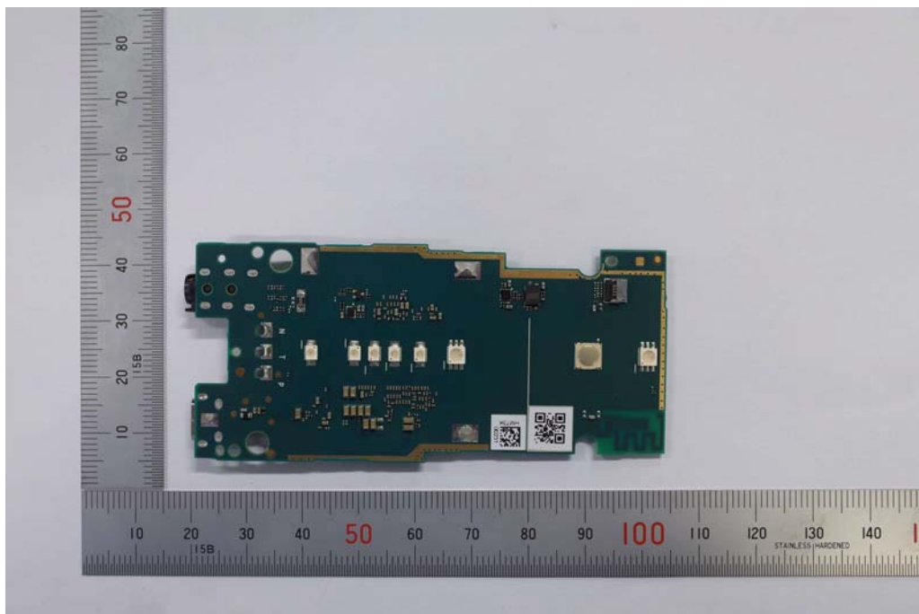
MAIN_bottom
