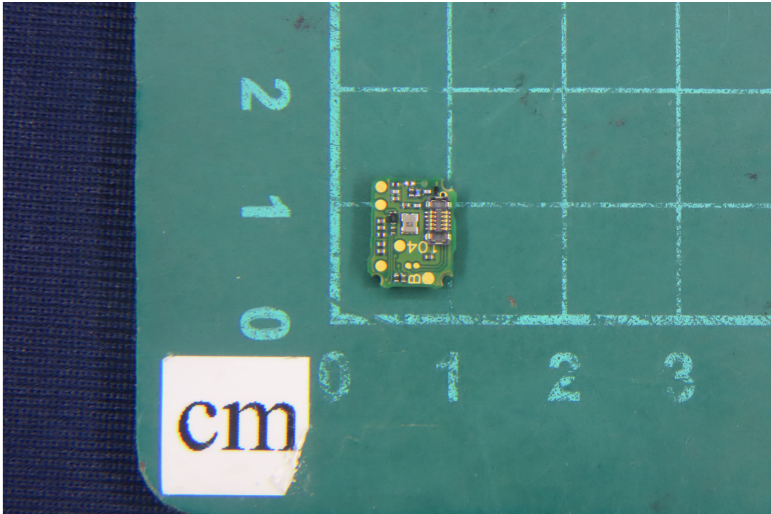
(19) EUT Photo
