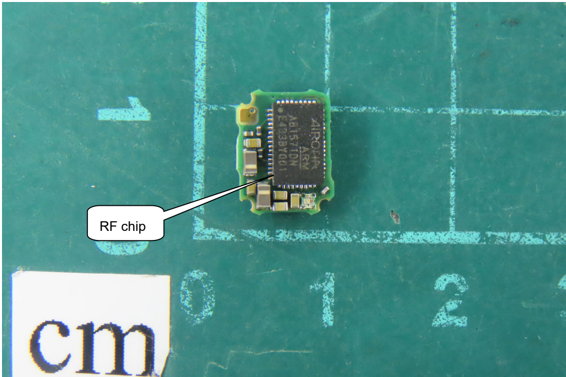
(18) EUT Photo
