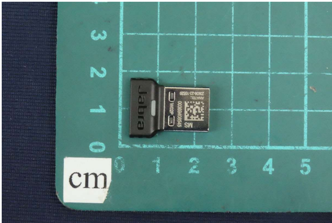
(2) EUT Photo
