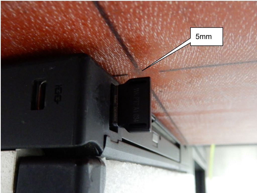
EUT Right-side(NB)
