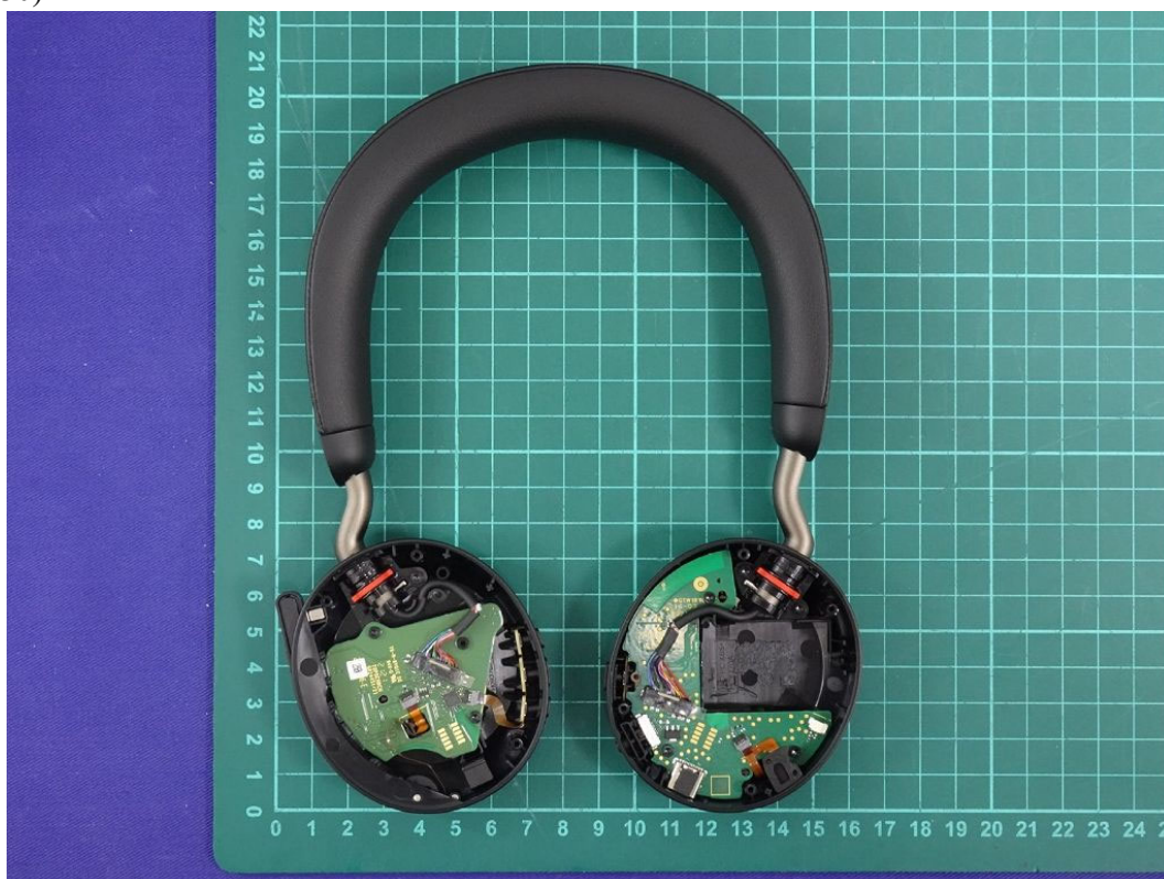
(30) EUT Photo
