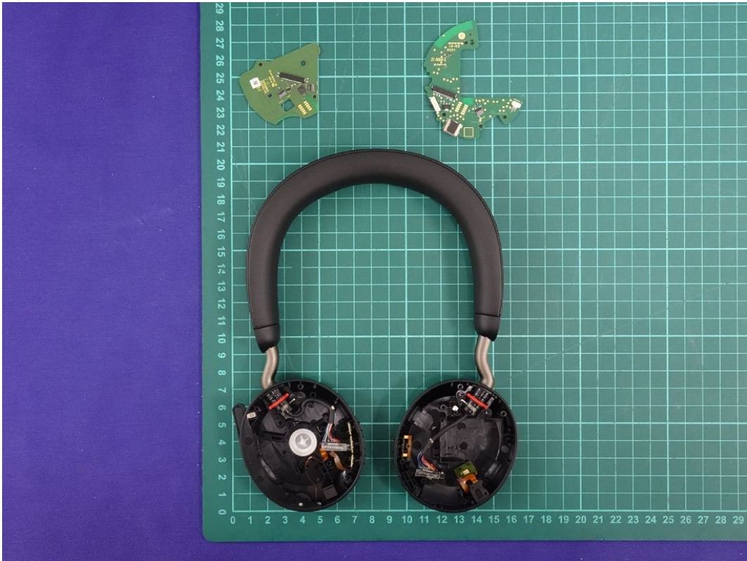
(31) EUT Photo
