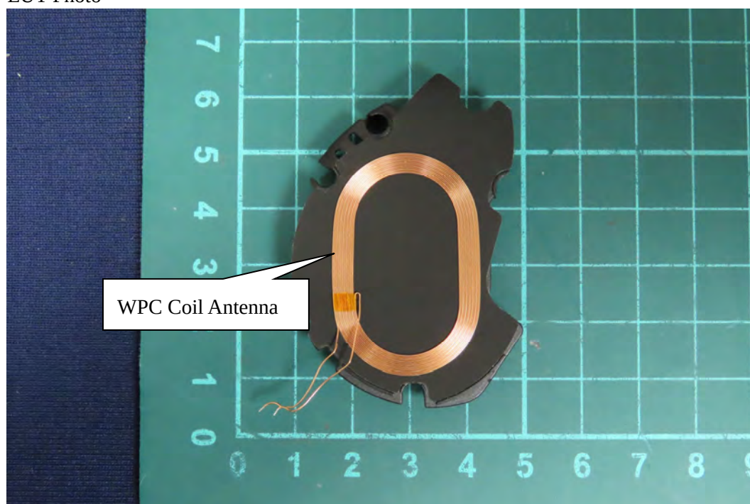
(21) EUT Photo
