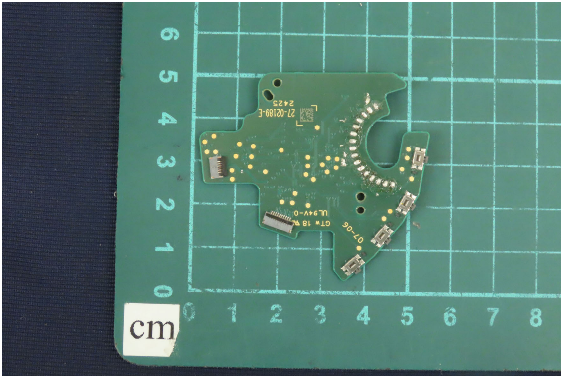
(17) EUT Photo
