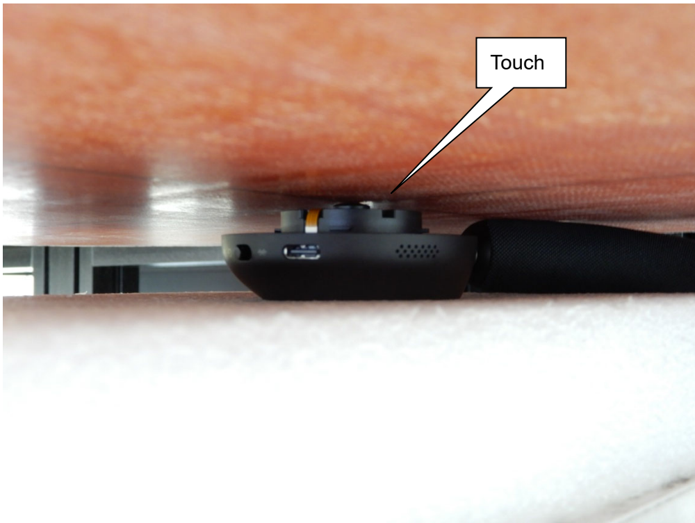
EUT Back
