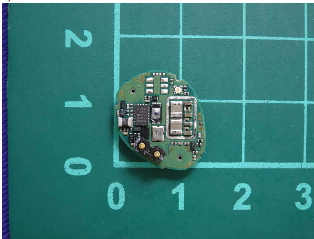
(56) EUT Photo
