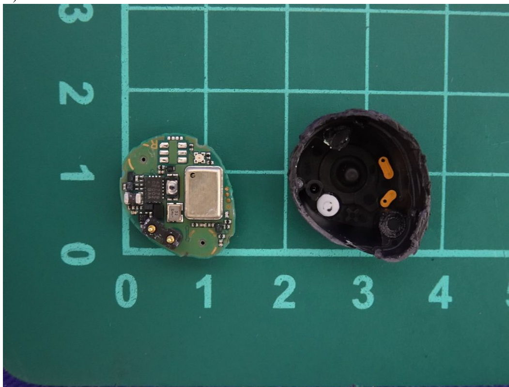
(53) EUT Photo
