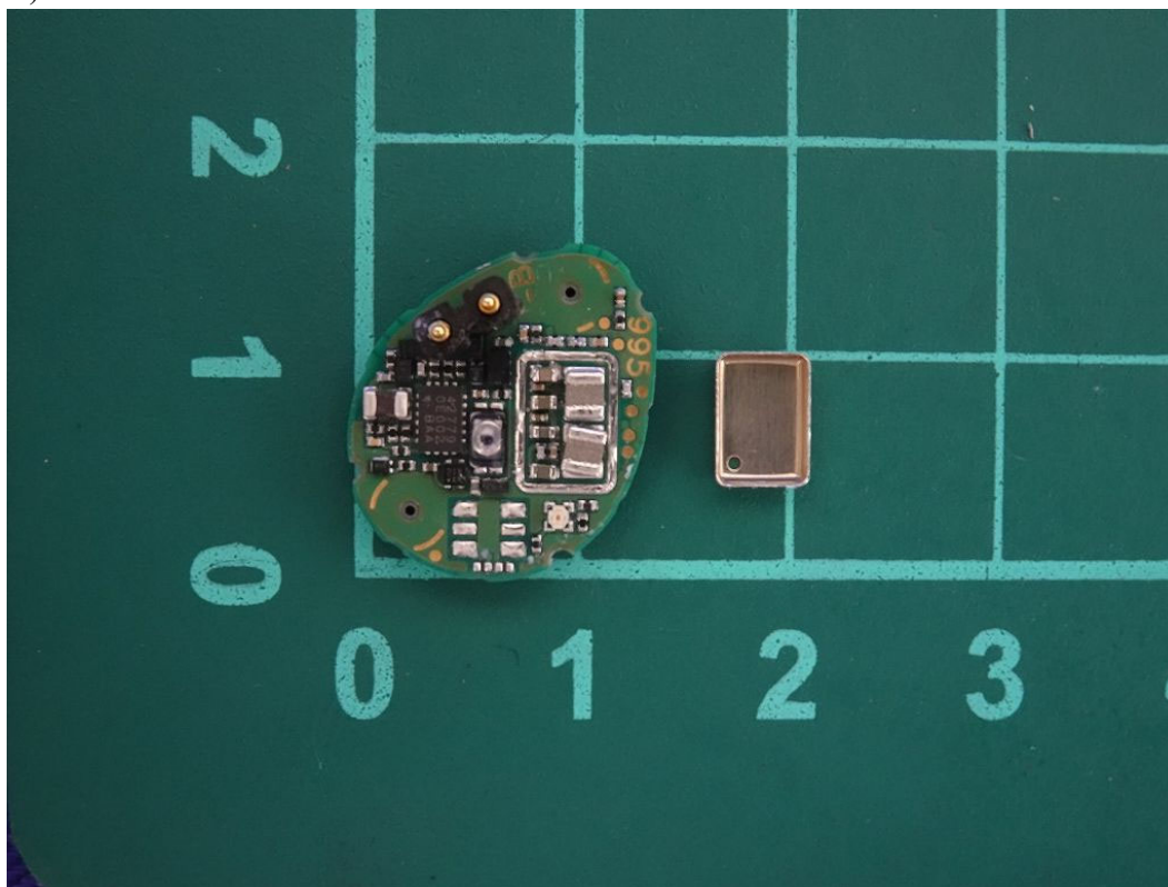
(66) EUT Photo
