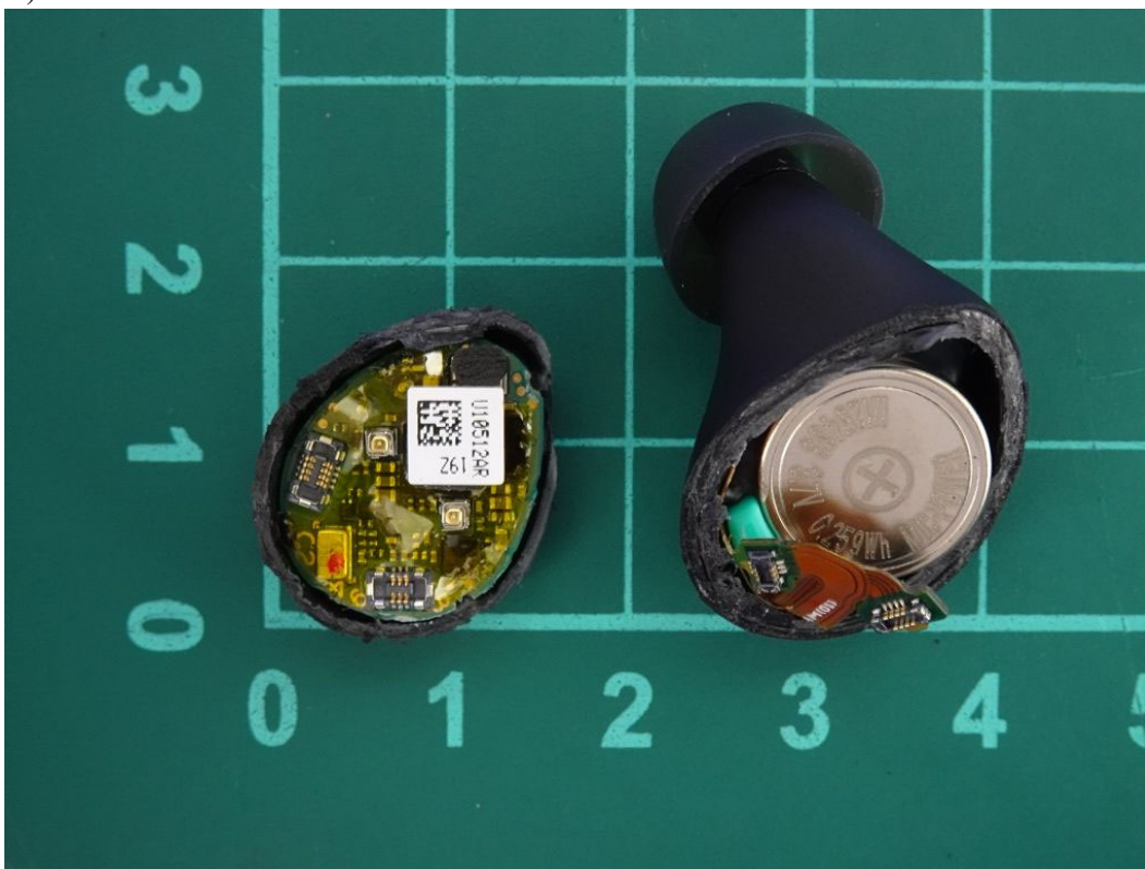
(50) EUT Photo
