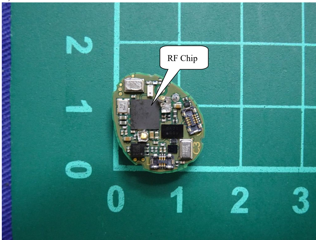
(46) EUT Photo
