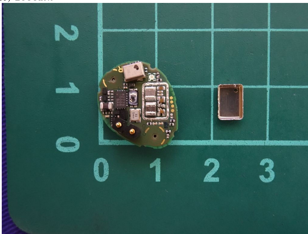
(33) EUT Photo
