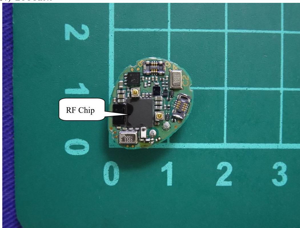
(57) EUT Photo
