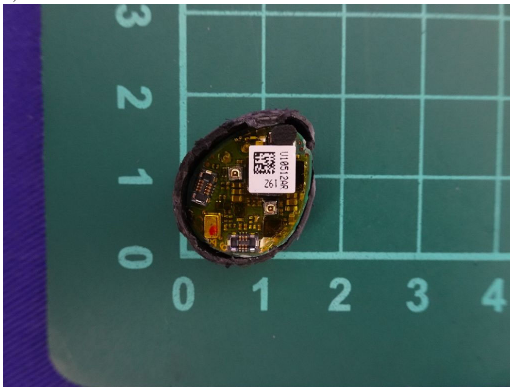
(52) EUT Photo
