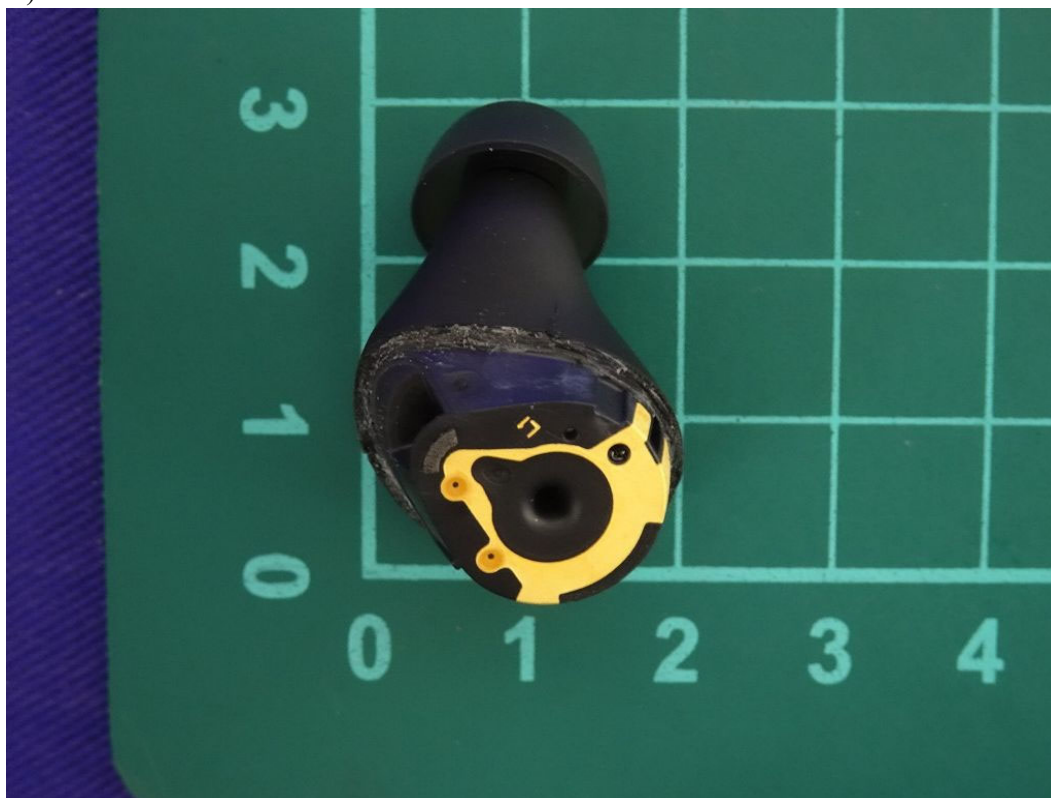
(59) EUT Photo
