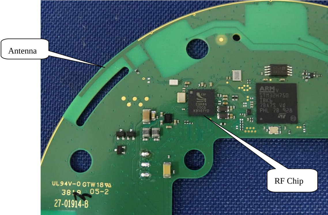
(14) EUT Photo
