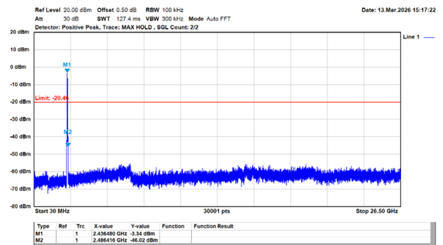
802.11ax/40MHz/MCS0/2452MHz/Ch9/Ant.1
