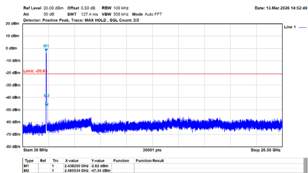
802.11ac/40MHz/MCS0/2452MHz/Ch9/Ant.1
