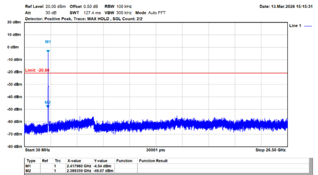
802.11ax/40MHz/MCS0/2437MHz/Ch6/Ant.1
