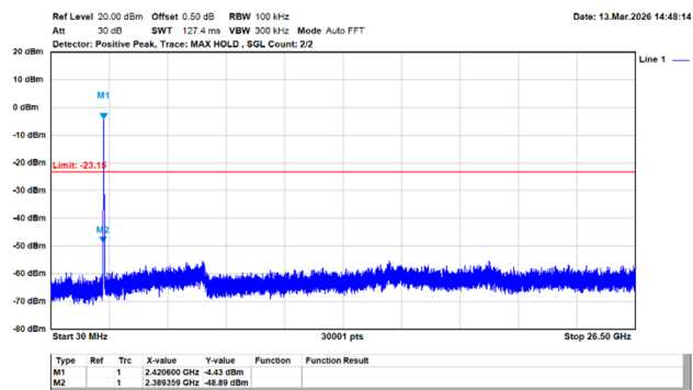
802.11ac/40MHz/MCS0/2437MHz/Ch6/Ant.1
