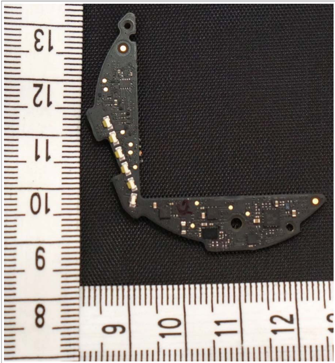
Right PCB
