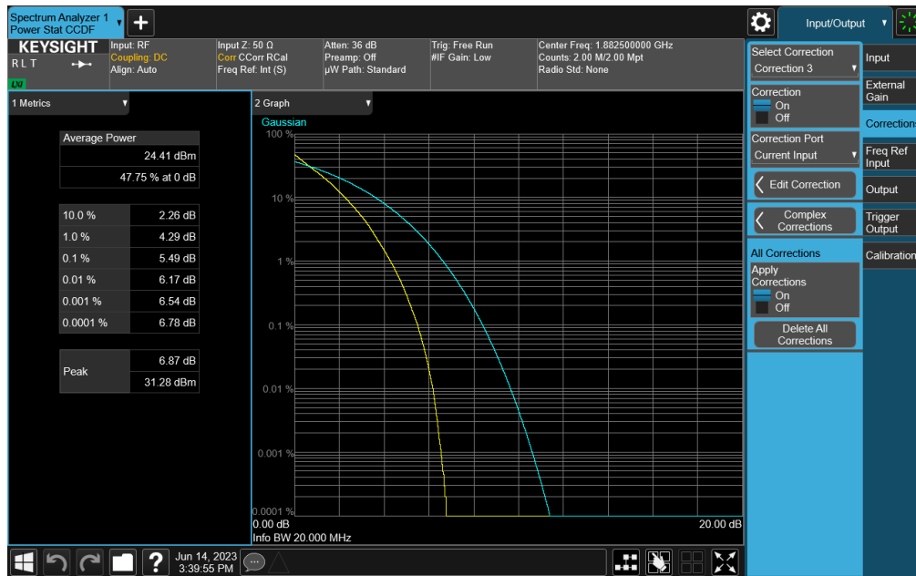
Plot 7-94. PAR Plot (LTE Band 25 - 20MHz QPSK - Full RB Configuration)
