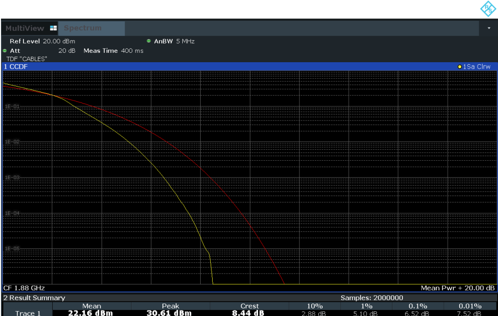
Plot 7-106. PAR Plot (LTE Band 2 - 5MHz QPSK - Full RB Configuration)
