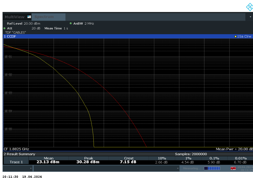
Plot 7-90. PAR Plot (LTE Band 25 - 1.4MHz QPSK - Full RB Configuration)
