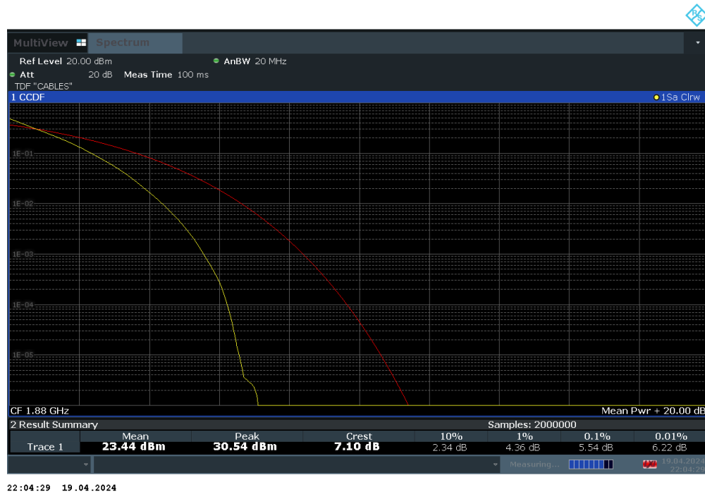
Plot 7-112. PAR Plot (LTE Band 2 - 20MHz QPSK - Full RB Configuration)
