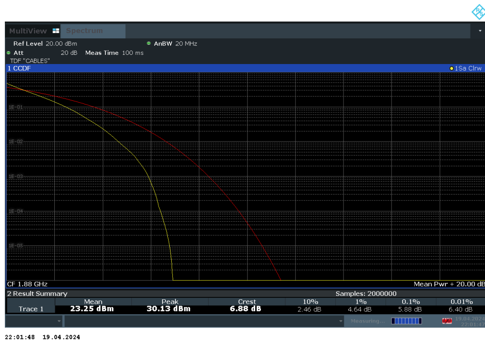
Plot 7-110. PAR Plot (LTE Band 2 - 15MHz QPSK - Full RB Configuration)
