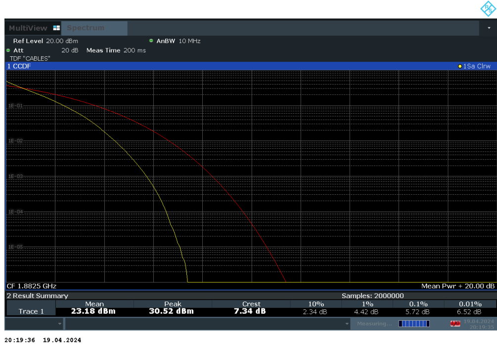
Plot 7-96. PAR Plot (LTE Band 25 - 10MHz QPSK - Full RB Configuration)
