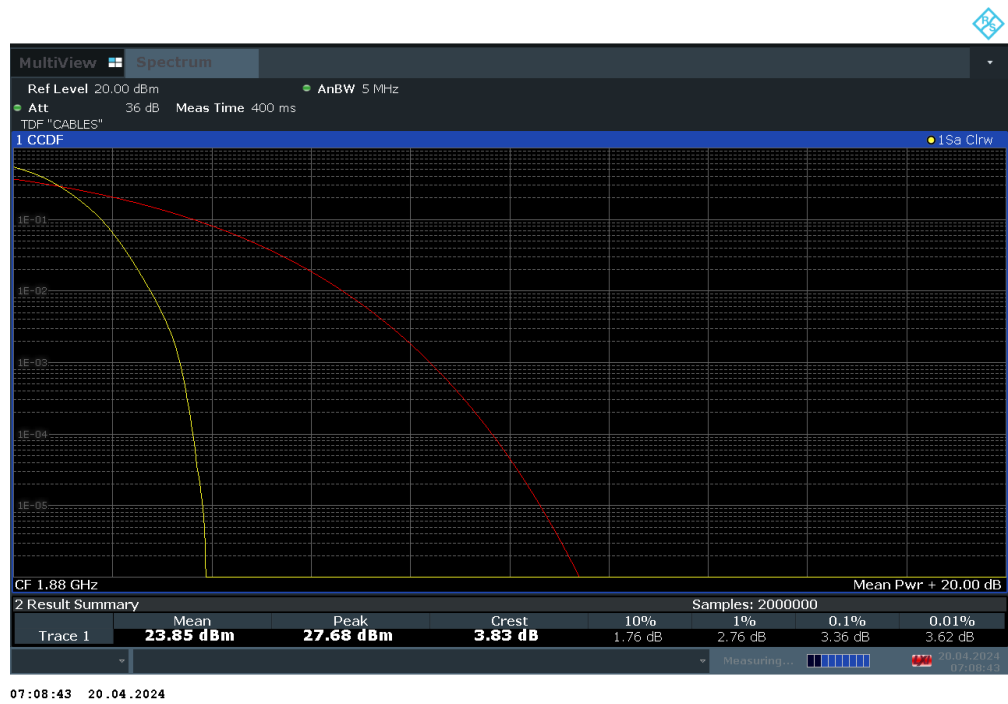
Plot 7-114. PAR Plot (WCDMA, Ch. 9400)
