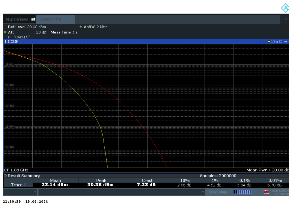
Plot 7-102. PAR Plot (LTE Band 2 - 1.4MHz QPSK - Full RB Configuration)
