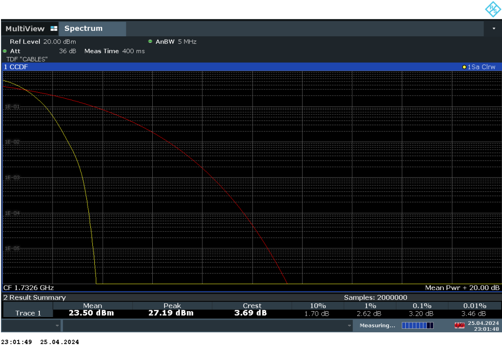
Plot 7-163. PAR Plot (WCDMA, Ch. 1413)
