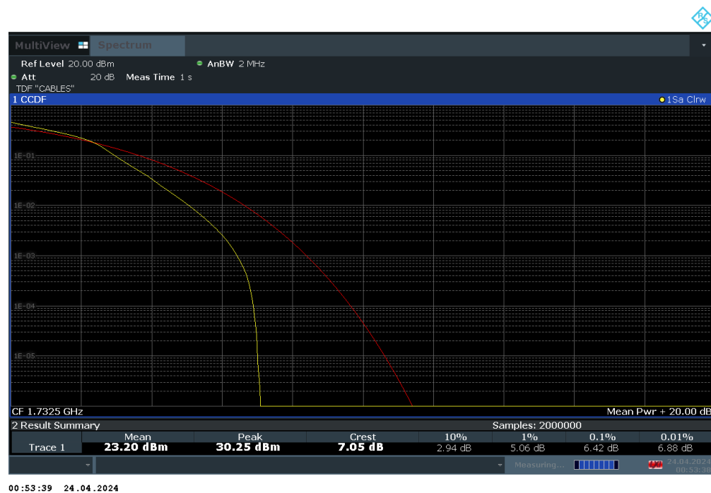
Plot 7-152. PAR Plot (LTE Band 4 - 1.4MHz 16-QAM - Full RB)
