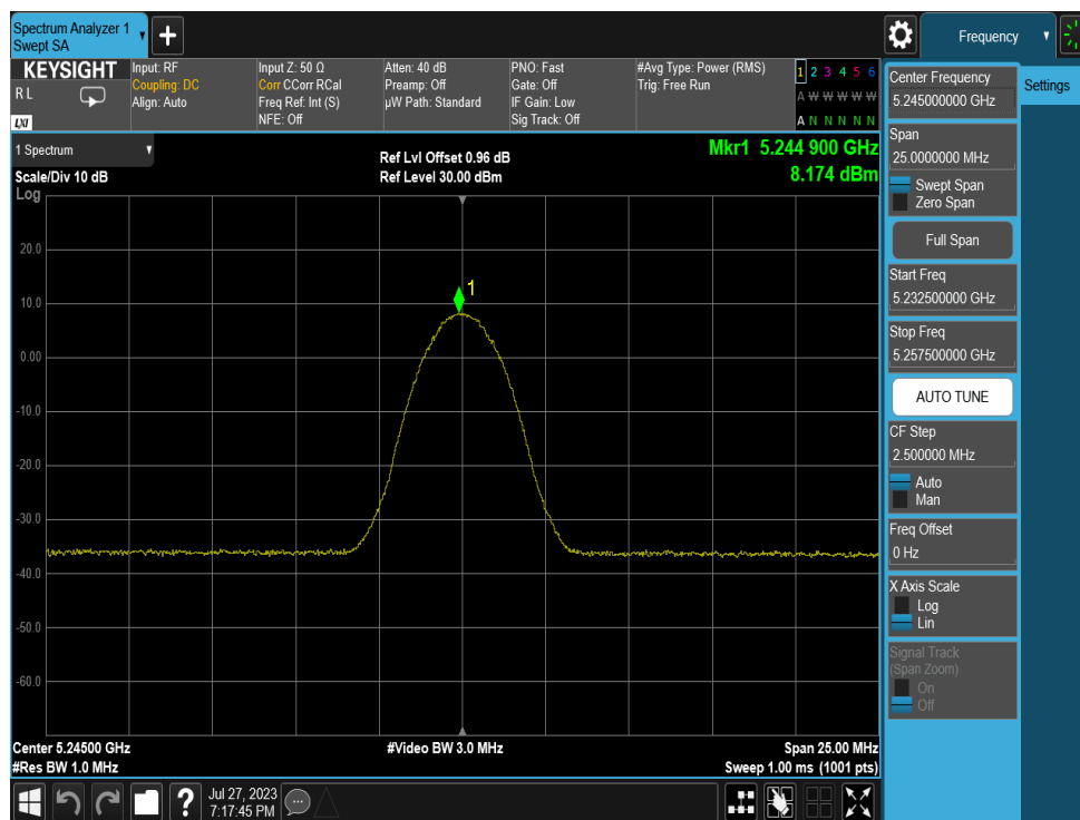
Plot 7-9. PSD (LE2M, 5245MHz)
