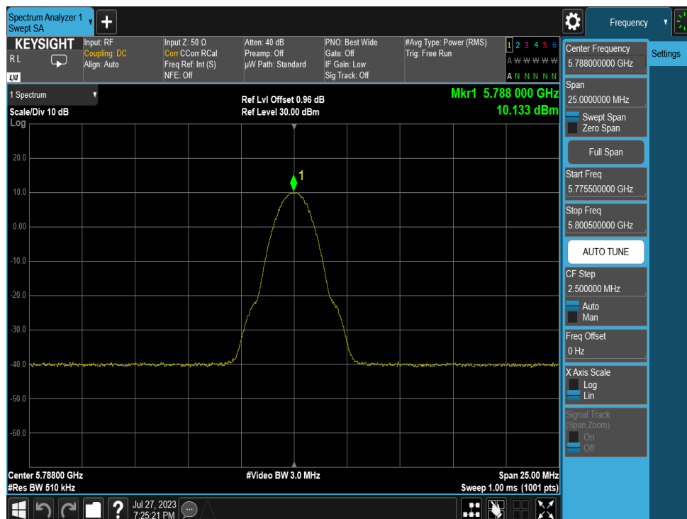
Plot 7-11. PSD (LE2M, 5788MHz)
