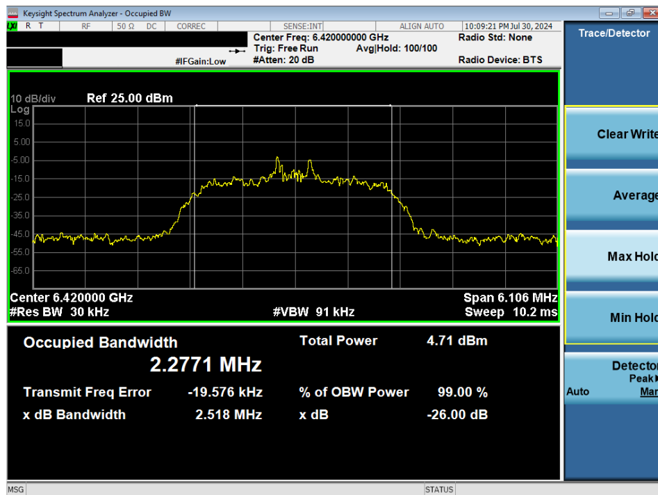
Plot 7-9. 26dB BW & 99% OBW (NB UNII HDR4 – 6420MHz)
