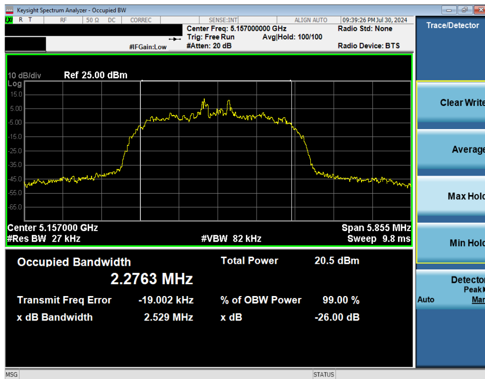
Plot 7-7. 26dB BW & 99% OBW (NB UNII HDR4 – 5157MHz)
