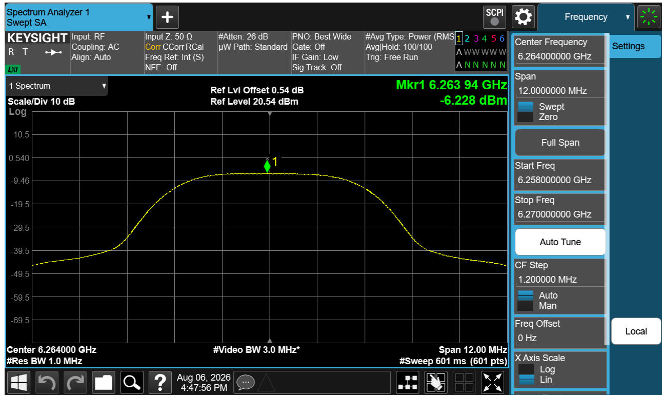
Plot 7-14. PSD (NB UNII HDRp8 - 6264MHz)
