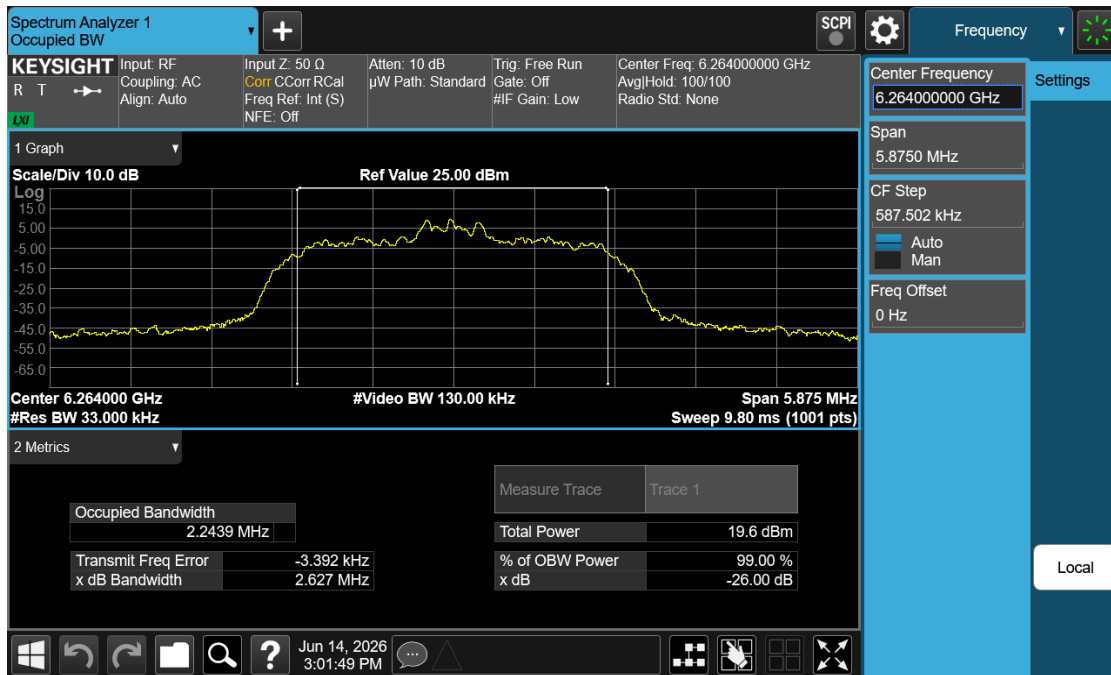
Plot 7-4. 26dB BW & 99% OBW (NB UNII HDR4 – 6264MHz)
