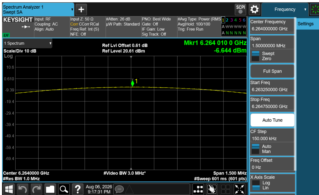
Plot 7-9. PSD (NB UNII LE1M – 6264MHz)
