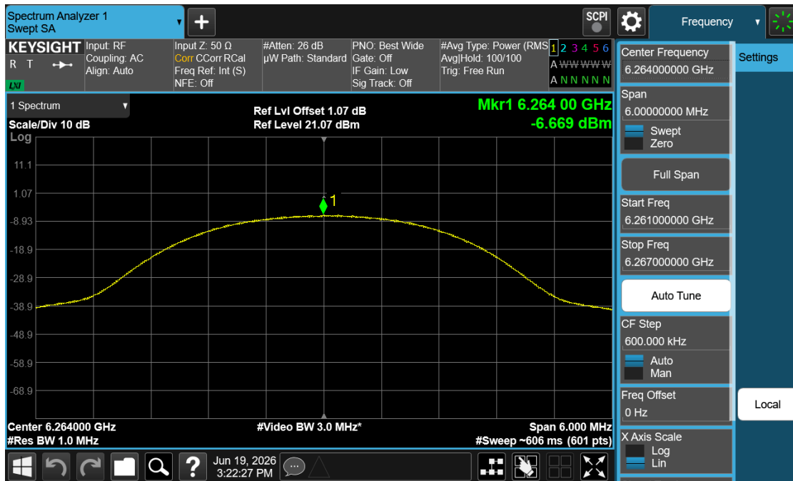
Plot 7-11. PSD (NB UNII HDR4 - 6264MHz)
