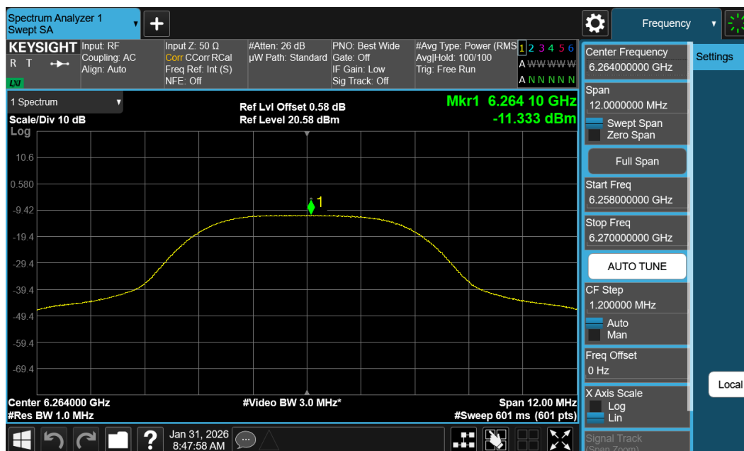
Plot 7-14. PSD (NB UNII HDRp8 – 6264MHz)
