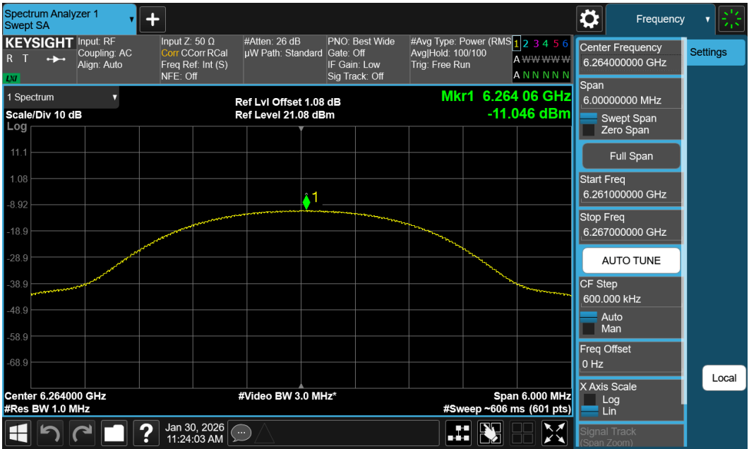
Plot 7-11. PSD (NB UNII HDR4 – 6264MHz)
