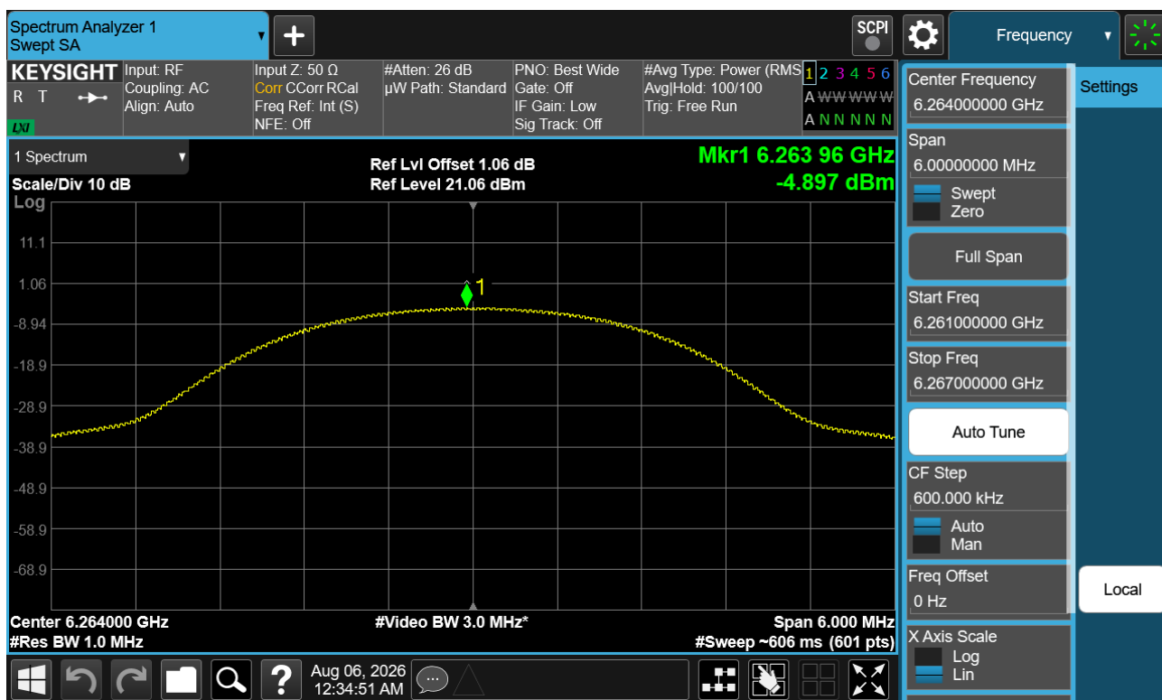
Plot 7-11. PSD (NB UNII HDR4 – 6264MHz)
