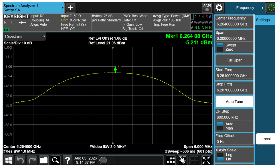
Plot 7-11. PSD (NB UNII HDR4 - 6264MHz)
