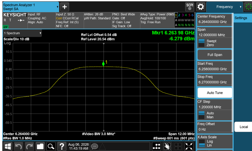
Plot 7-14. PSD (NB UNII HDRp8 – 6264MHz)
