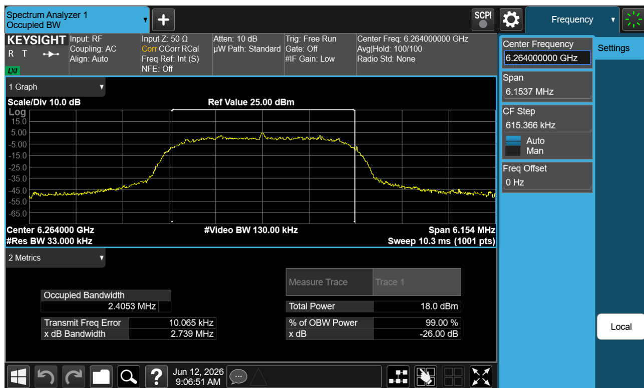
Plot 7-6. 26dB BW & 99% OBW (NB UNII HDRp4 – 6264MHz)
