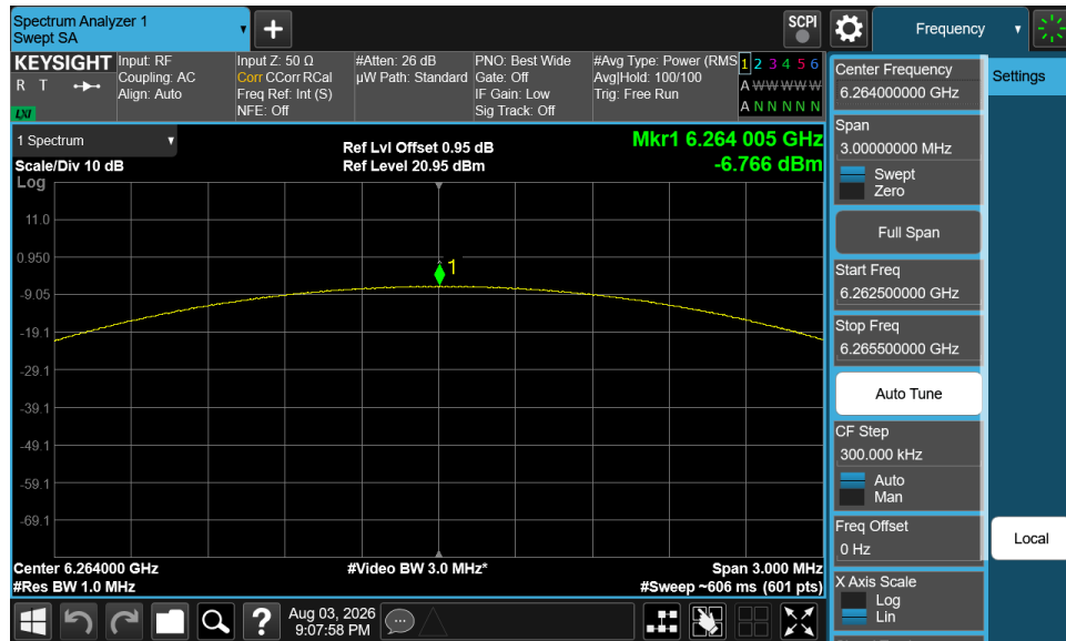
Plot 7-10. PSD (NB UNII LE2M - 6264MHz)
