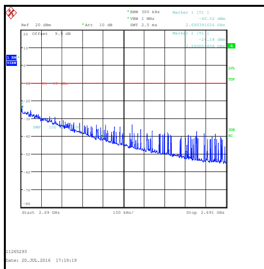
QPSK / 1 RB 74 Offset / Upper Band Edge
