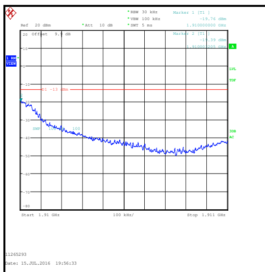
16QAM / 1 RB 14 offset / Upper Band Edge
