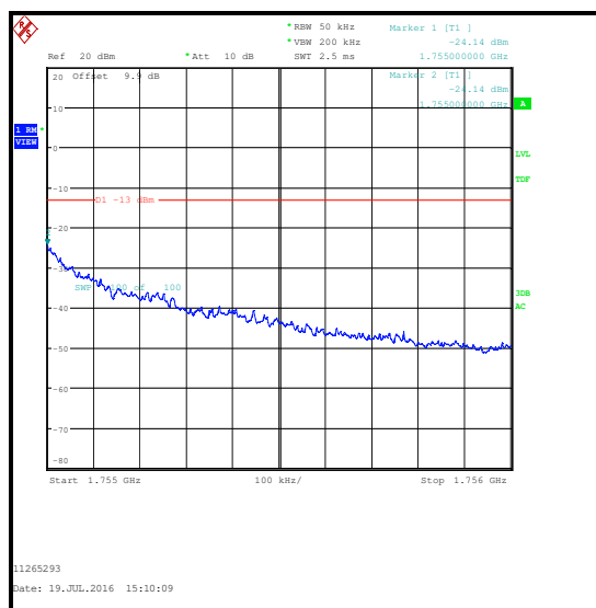
QPSK / 1 RB 24 offset / Upper Band Edge
