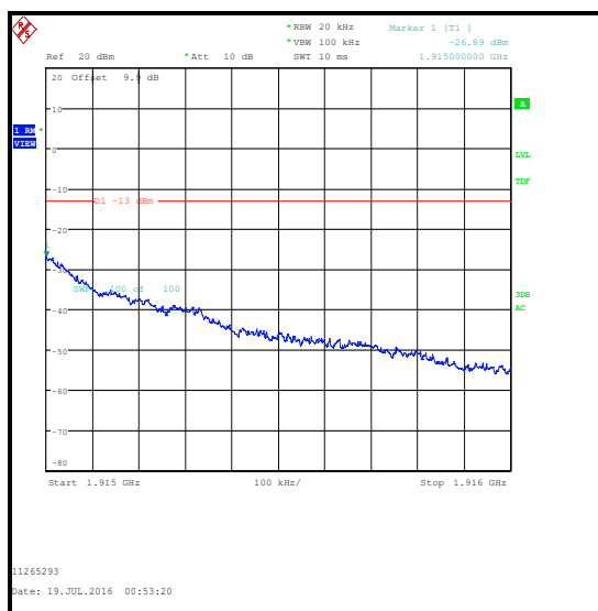
QPSK / 1 RB 5 offset / Upper Band Edge
