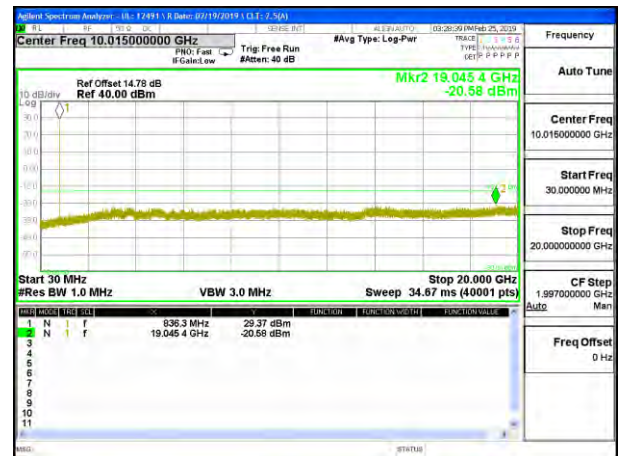
GSM 850MHz EGPRS Middle Channel
