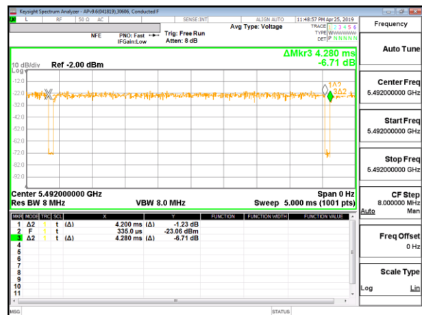
802.11ax HE80 1TX, 26-TONES
