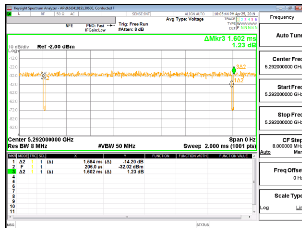
802.11ax HE40 OFDMA, 484-TONES
