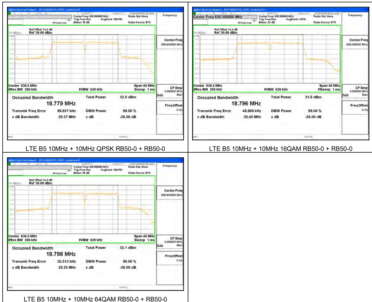
LTE B5 10MHz + 10MHz 64QAM RB50-0 + RB50-0
