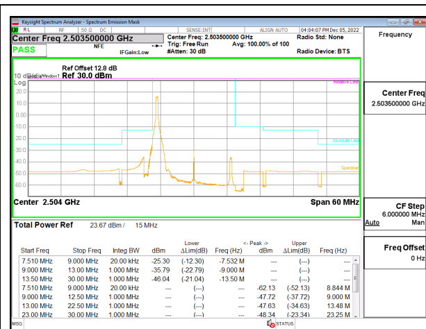
5G NR n41 15MHz BPSK Low Channel RB1-0 ID:28498
