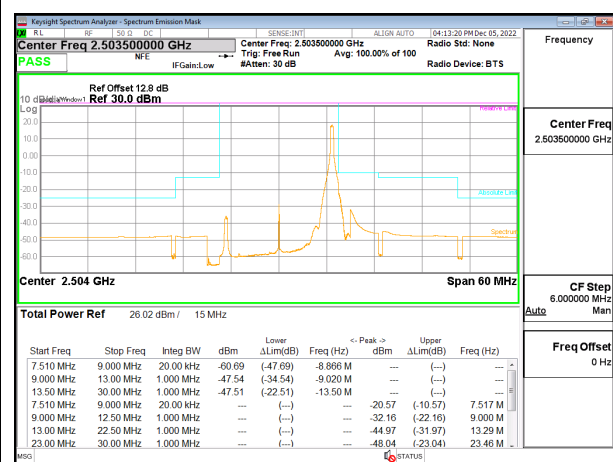
5G NR n41 15MHz BPSK Low Channel RB1-37 ID:28498
