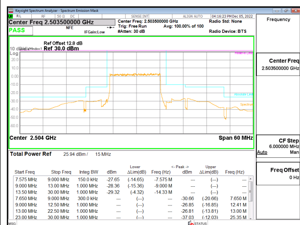
5G NR n41 15MHz BPSK Low Channel RB36-0 ID:28498
