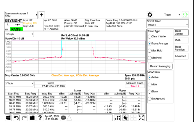
5G NR n77 30MHz BPSK Mid Channel RB75-0 Port B ID 27342
