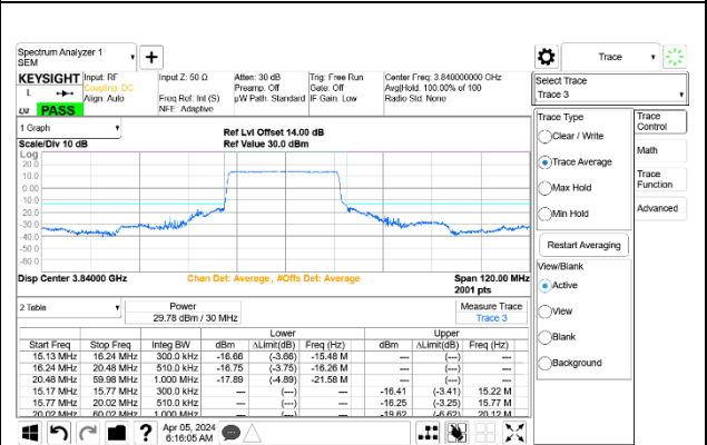
5G NR n77 BPSK BPSK Mid Channel RB75-0 Port A+B ID 27342
