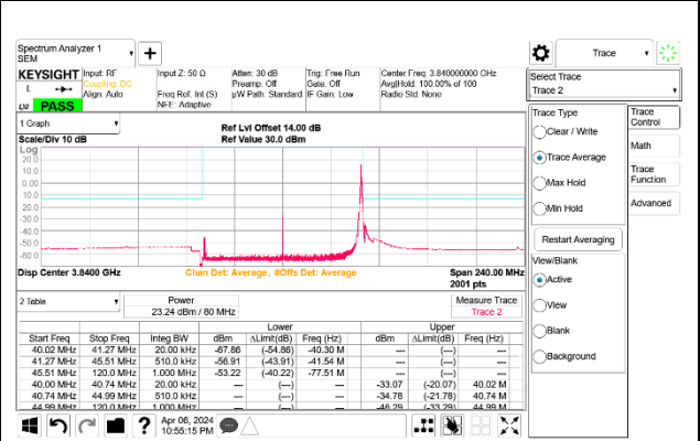
5G NR n77 80MHz BPSK Mid Channel RB1-216 Port B
