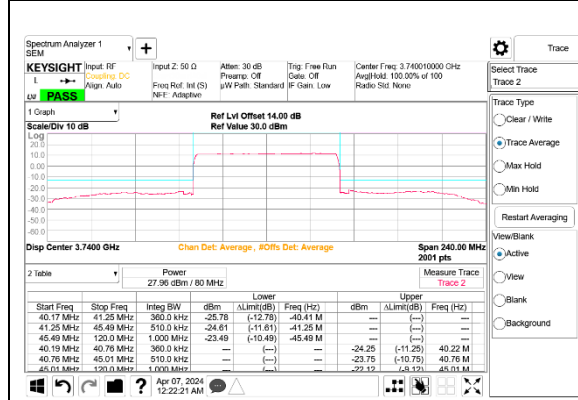
5G NR n77 80MHz BPSK Low Channel RB216-0 Port B
