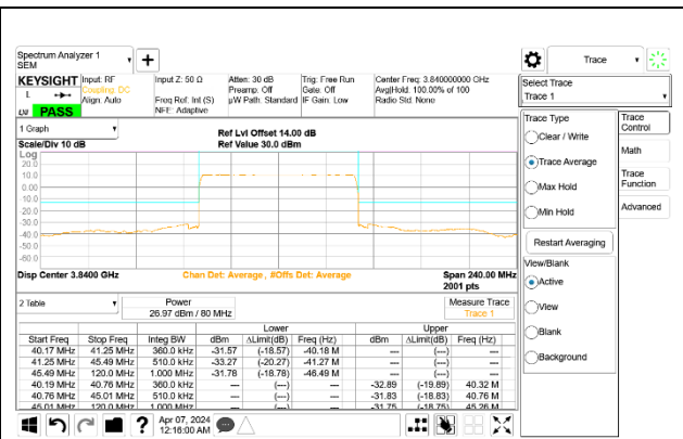
5G NR n77 80MHz BPSK Mid Channel RB216 -0 Port A
