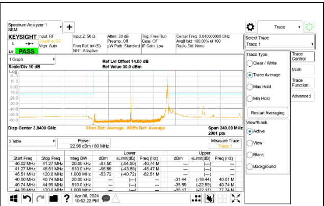
5G NR n77 80MHz BPSK Mid Channel RB1-216 Port A
