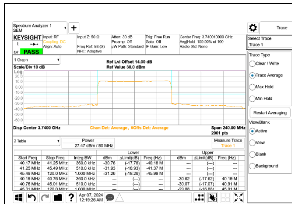
5G NR n77 80MHz BPSK Low Channel RB216 -0 Port A
