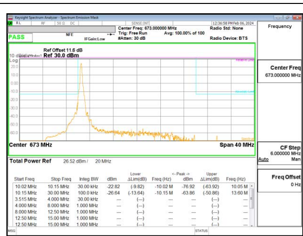
5G NR n71 20MHz BPSK Low Channel RB1-0, ID:28567
