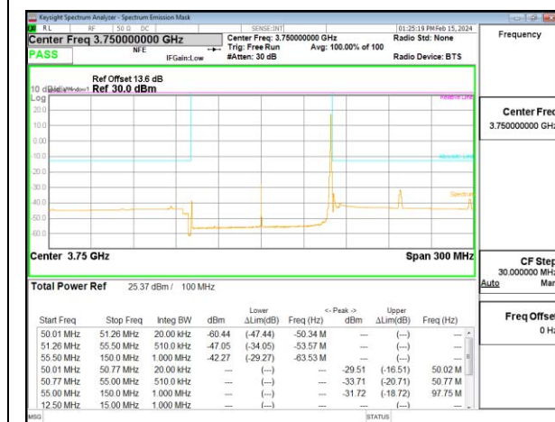
5G NR n77 100MHz BPSK Low Channel RB1-272, ID:28567
