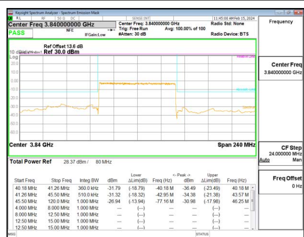
5G NR n77 80MHz BPSK Middle Channel RB216-0, ID:28567
