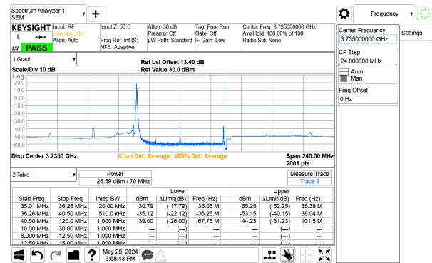
5G NR n77 70MHz BPSK Low Channel RB1-0 Port A+B ID: 32546
