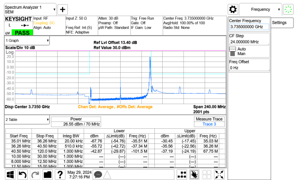
5G NR n77 70MHz BPSK Low Channel RB1-188 Port A+B ID: 32546
