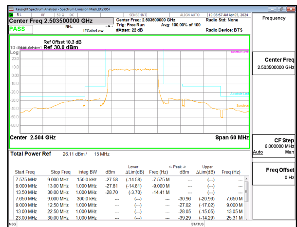
5G NR n41 15MHz BPSK Low Channel RB36-0
