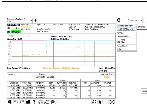
5G NR n66 20MHz BPSK Low Channel RB100-0 ID:28498
