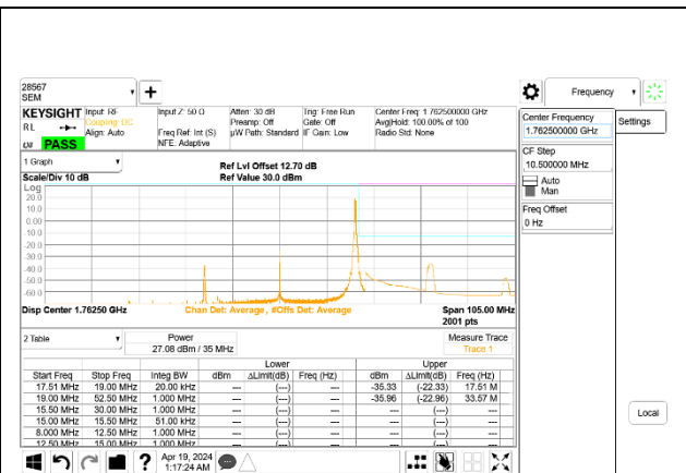
5G NR n66 35MHz BPSK High Channel RB1-187
