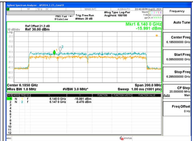
TPC PSD CH47@ 6185-160MHz – ANT 5
