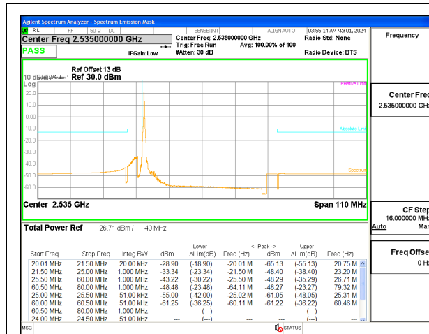
5G NR n7 40MHz BPSK Middle Channel RB1-0, ID:12482
