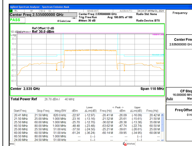
5G NR n7 40MHz BPSK Middle Channel RB216-0, ID:12482
