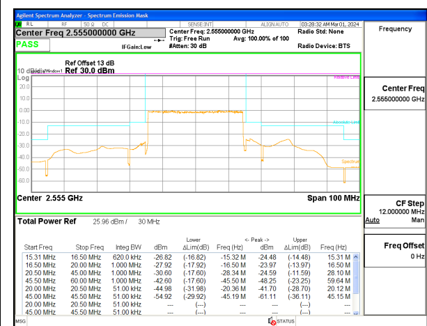
5G NR n7 30MHz BPSK High Channel RB160-0, ID:12482
