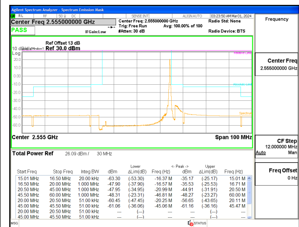
5G NR n7 30MHz BPSK High Channel RB1-159, ID:12482
