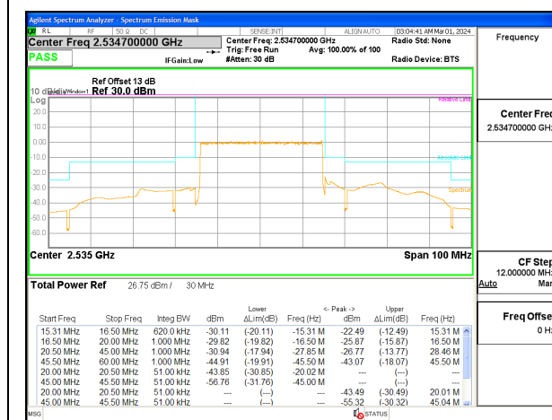
5G NR n7 30MHz BPSK Middle Channel RB160-0, ID:12482
