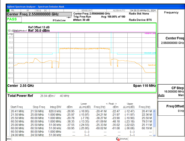
5G NR n7 40MHz BPSK High Channel RB216-0, ID:12482
