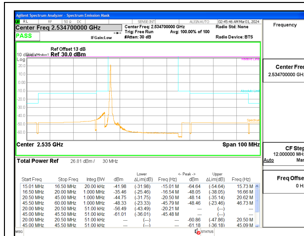
5G NR n7 30MHz BPSK Middle Channel RB1-0, ID:12482
