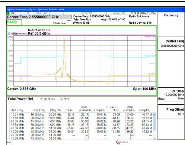
5G NR n7 30MHz BPSK High Channel RB1-0, ID:12482
