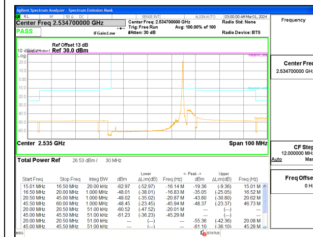
5G NR n7 30MHz BPSK Middle Channel RB1-159, ID:12482
