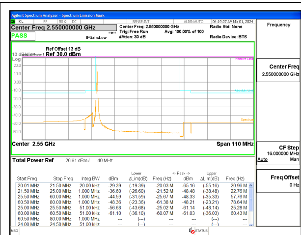
5G NR n7 40MHz BPSK High Channel RB1-0, ID:12482
